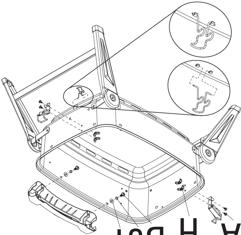
Acople los seguros y la bisagra
